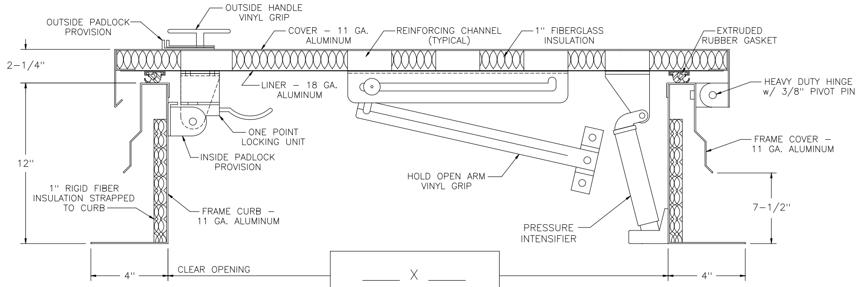
SECTION A-A
